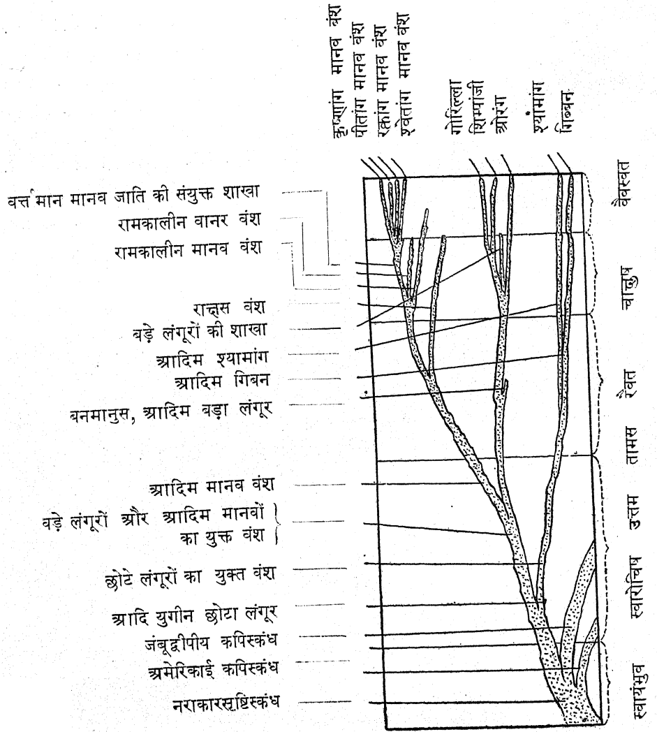
चित्र १४—नराकार प्राणियों का क्रमविकास-वृत्त
